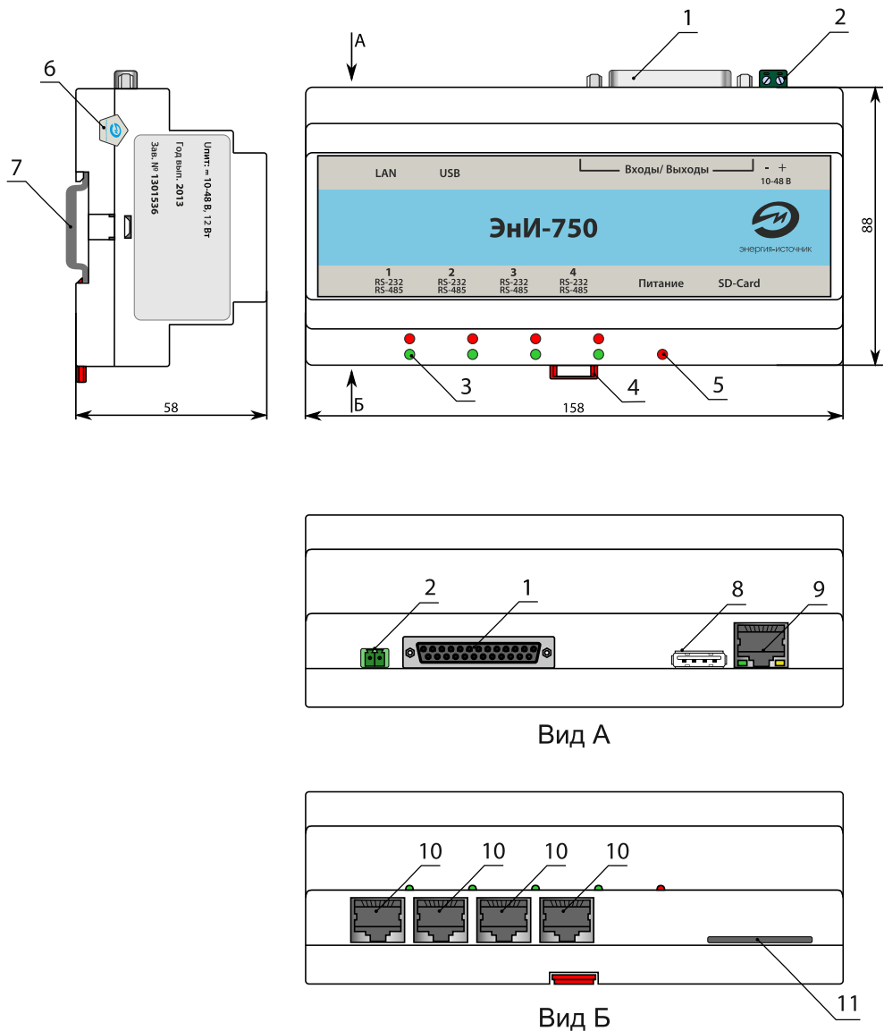
Рисунок 2. Внешний вид ПЛК
