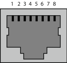
Рисунок А.3. Вид разъема интерфейсов RS-232 / RS-485 Таблица А.4. Назначение выводов разъемов RS-232 / RS-485
