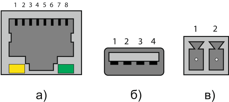
Рисунок А.1. Вид разъемов: а) Ethernet; б) USB; в) питание Таблица А.1. Назначение выводов разъема Ethernet
