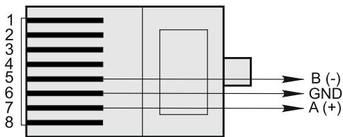
Рисунок В.2. Кабель связи ПЛК по интерфейсу RS-485
