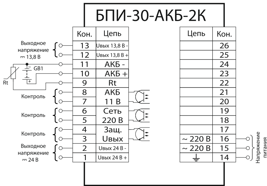
Рисунок В.1. Схема подключения блока
