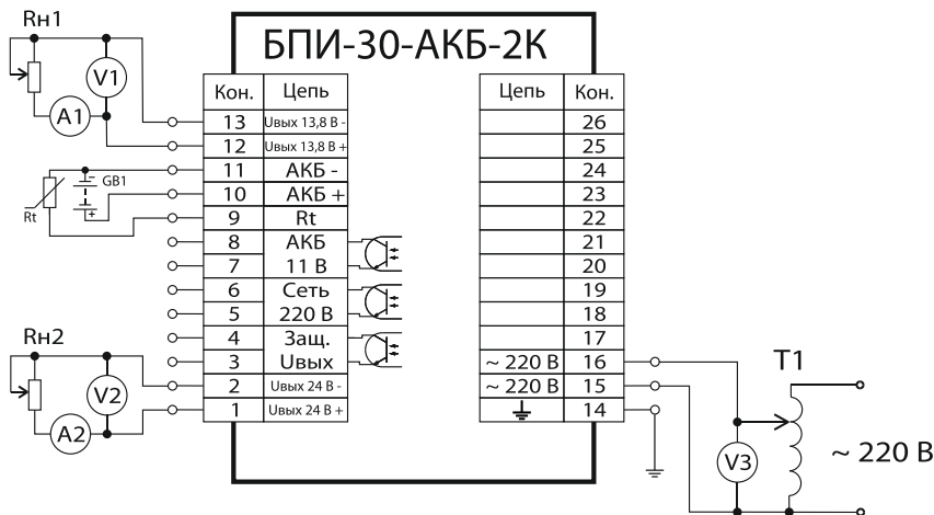
Рисунок Г.1. Схема проверки нагрузочной способности блока
