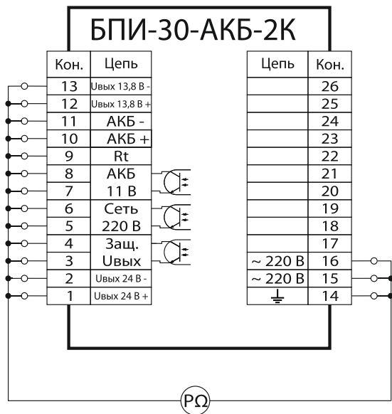
Рисунок Г.2. Схема проверки сопротивления изоляции блока — PΩ – мегаомметр.
