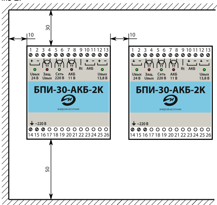
Рисунок 2. Установка блока
