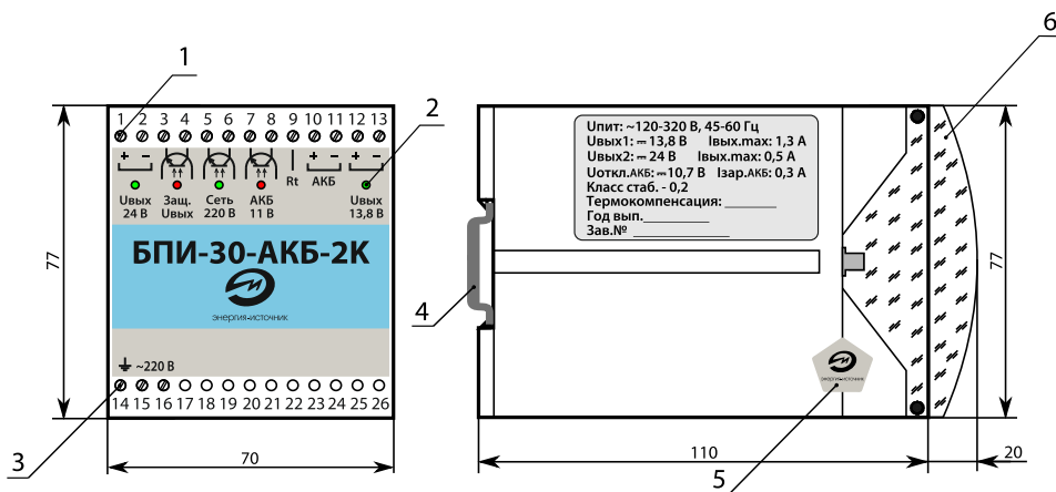
Рисунок Б.1. Габаритные размеры блока
