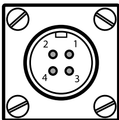
Рисунок Б.3. Нумерация контактов разъемов XP1, для подключения напряжения питания (исполнение 01Р, 01К) и XP2, XP3 для подключения выходных цепей (исполнение 01Р)
