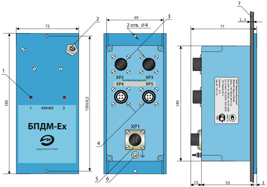
Рисунок Б.4. Габаритные размеры блока (исполнение 01P)
