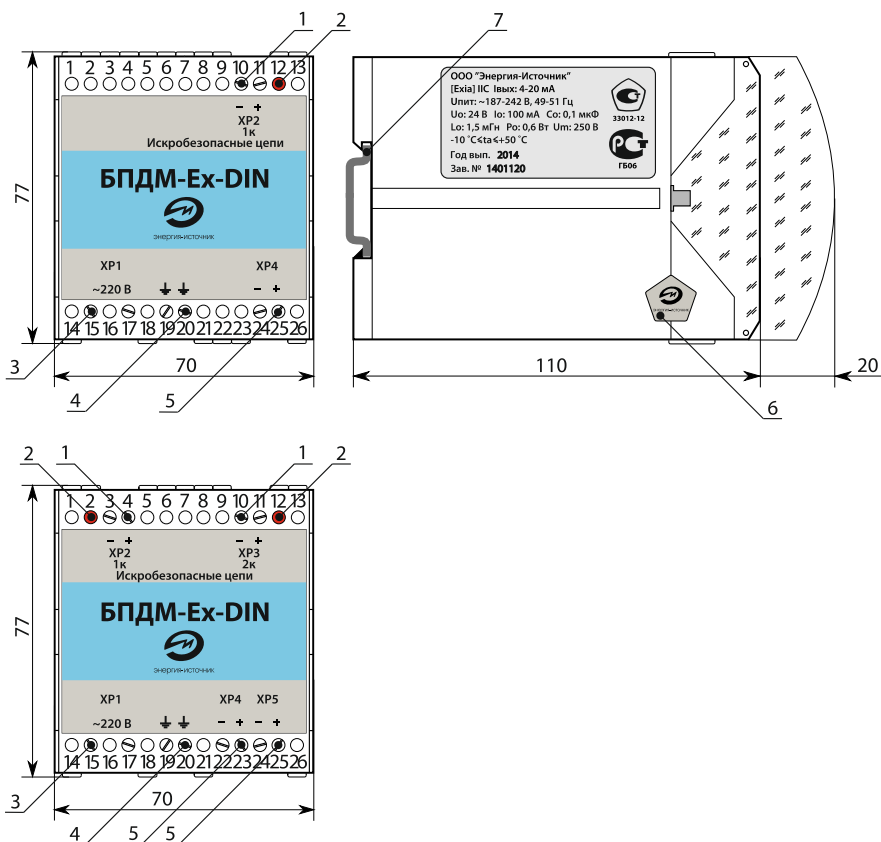
Рисунок Б.1. Габаритные размеры блока (исполнение DIN)
