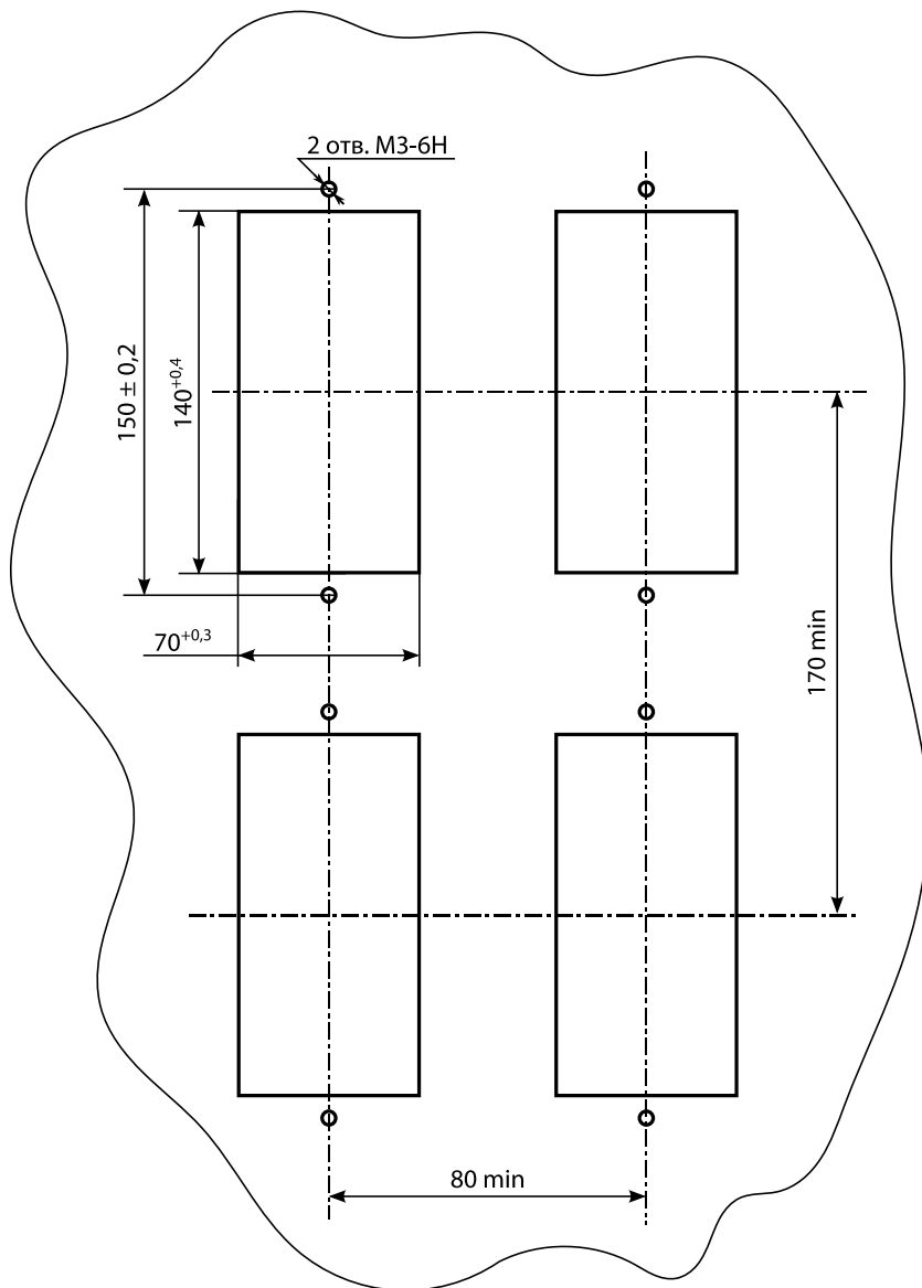
Рисунок Б.6. Разметка под вырезы в щите (исполнение 01Р, 01К)
