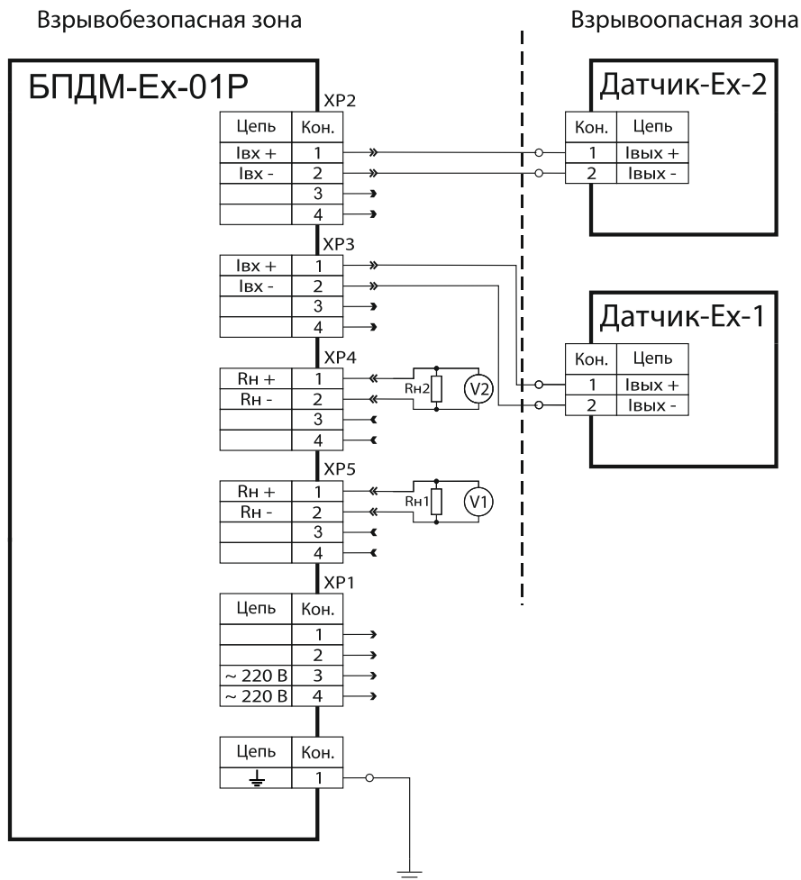
Рисунок В.3. Схема подключения блока (исполнение 01Р)
