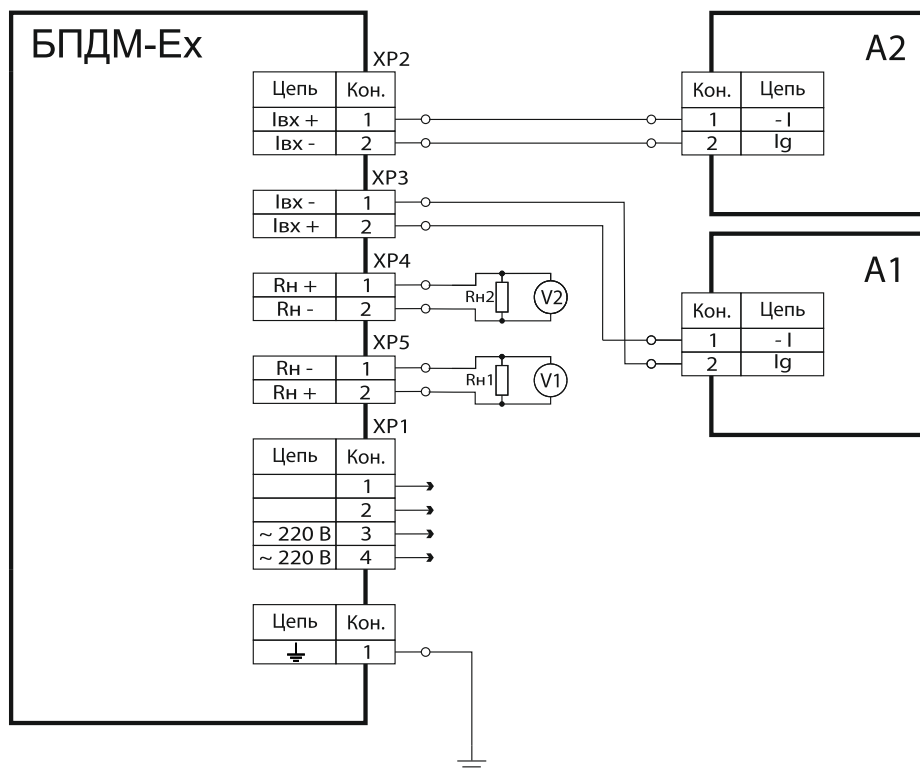
Рисунок Г.1. Схема поверки блока
