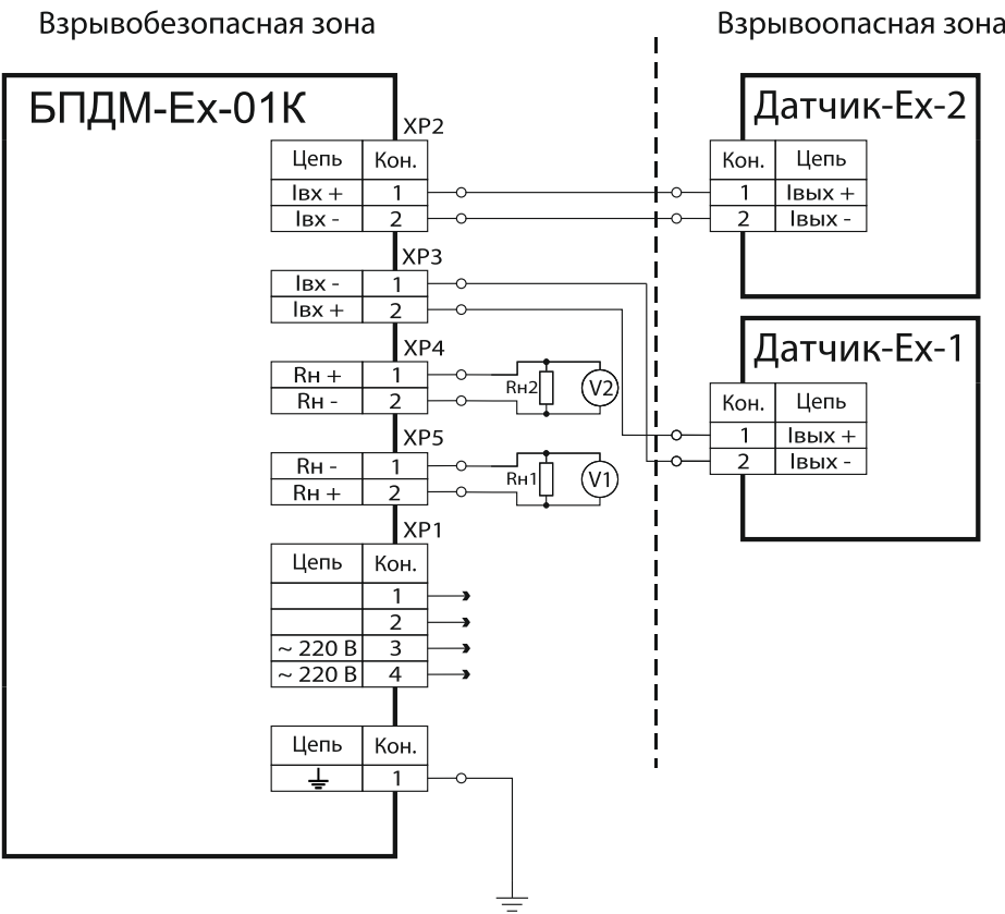
Рисунок В.2. Схема подключения блока (исполнение 01К)
