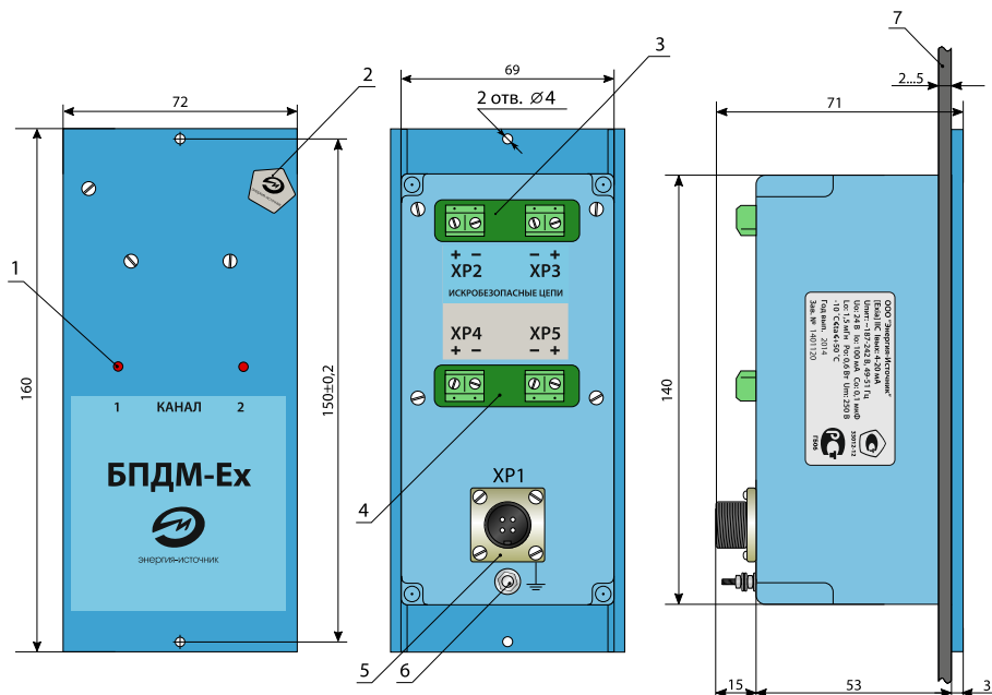
Рисунок Б.2. Габаритные размеры блока (исполнение 01К)
