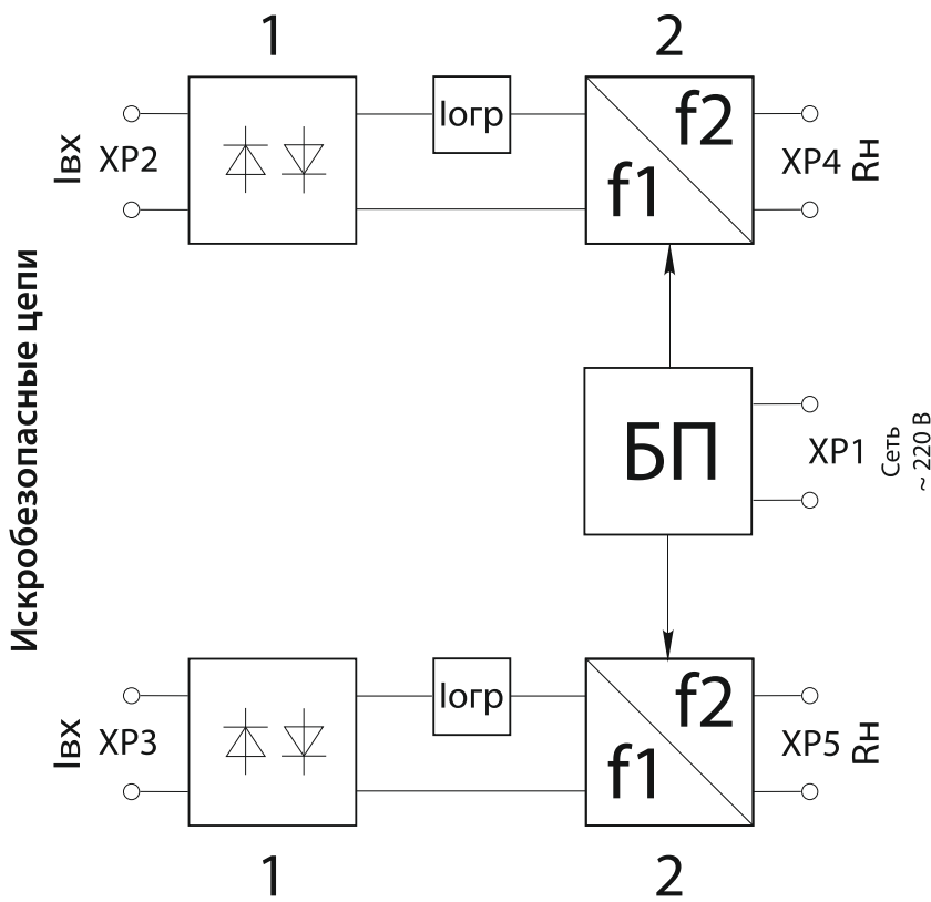
Рисунок А.1. Функциональная схема блока
