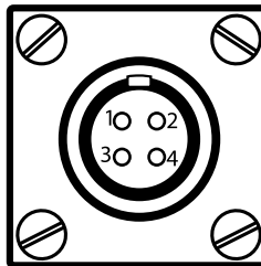
Рисунок Б.5. Нумерация контактов разъемов XP4,XP5 для подключения выходных цепей (исполнение 01P)
