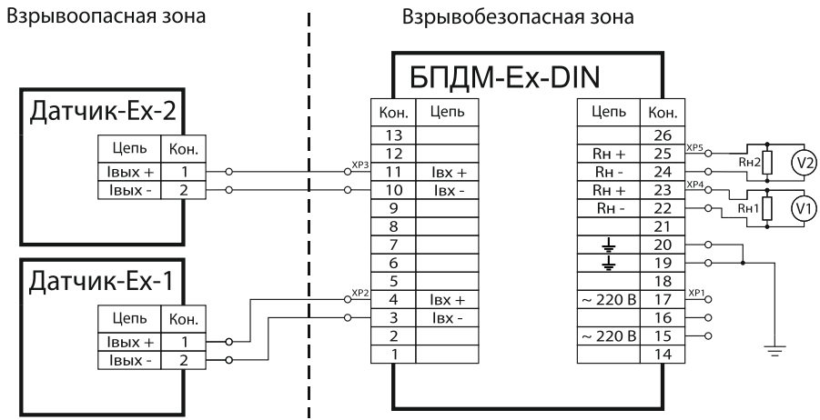
Рисунок В.1. Схема подключения блока (исполнение DIN)
