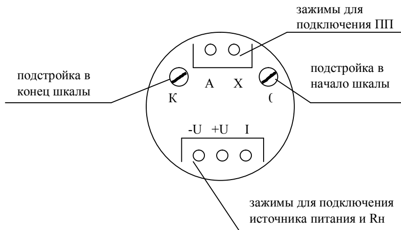
Рис.4. Расположение, маркировка и назначение органов управления и зажимов для ПИ диапазона сигналов 0...5 мА и ПП типа ТХА.
